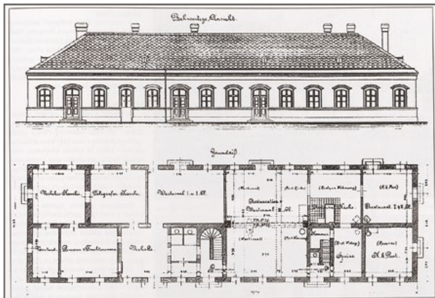
Plán nádražní budovy v Tlumačově a Rohatci.
