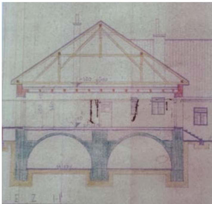
Řez budovou pivovaru, ve kterém jsou vidět sklepy
